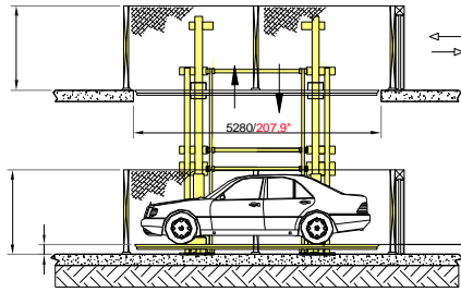
L - GD
